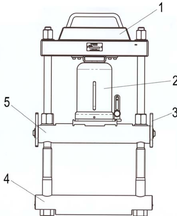
Figura 1: Conjunto general estrangulador hidráulico
