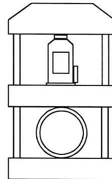
Figura 8: Posicionado del tubo correcto
